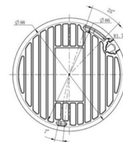
AI IR Mini Dome Network Camera | Dimensions
