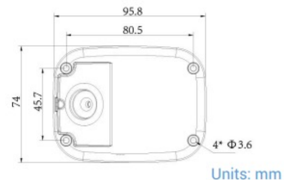
AI 180° Panoramic Mini Bullet Network Camera | Dimensions
